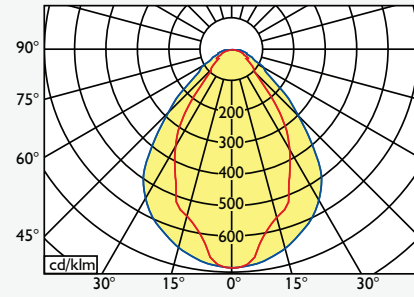
MPRM — C0-C180 — C90-C270
