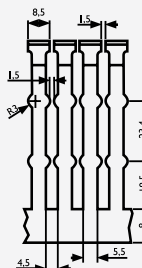
Bauhöhe 80
