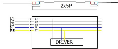
Anschluss / Connection 2x5P
